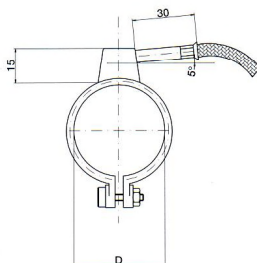
Tangenziale a 5° Tangential 5°
