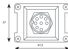
Connettore M 12 a 8 poli
