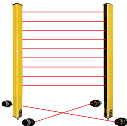
Versione a 2 sensori incrociati
