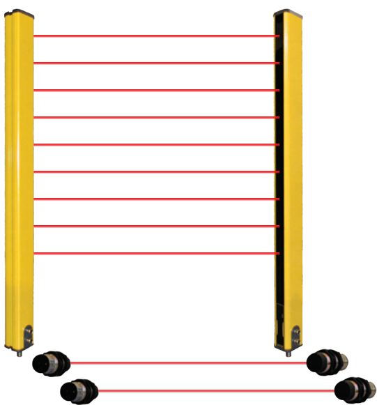
Versione a 2 sensori paralleli
